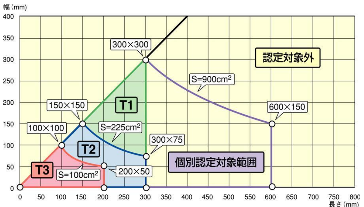
図 1 型式（T1～T3）の範囲とその他の範囲（長さ及び幅及び面積(S)について）
